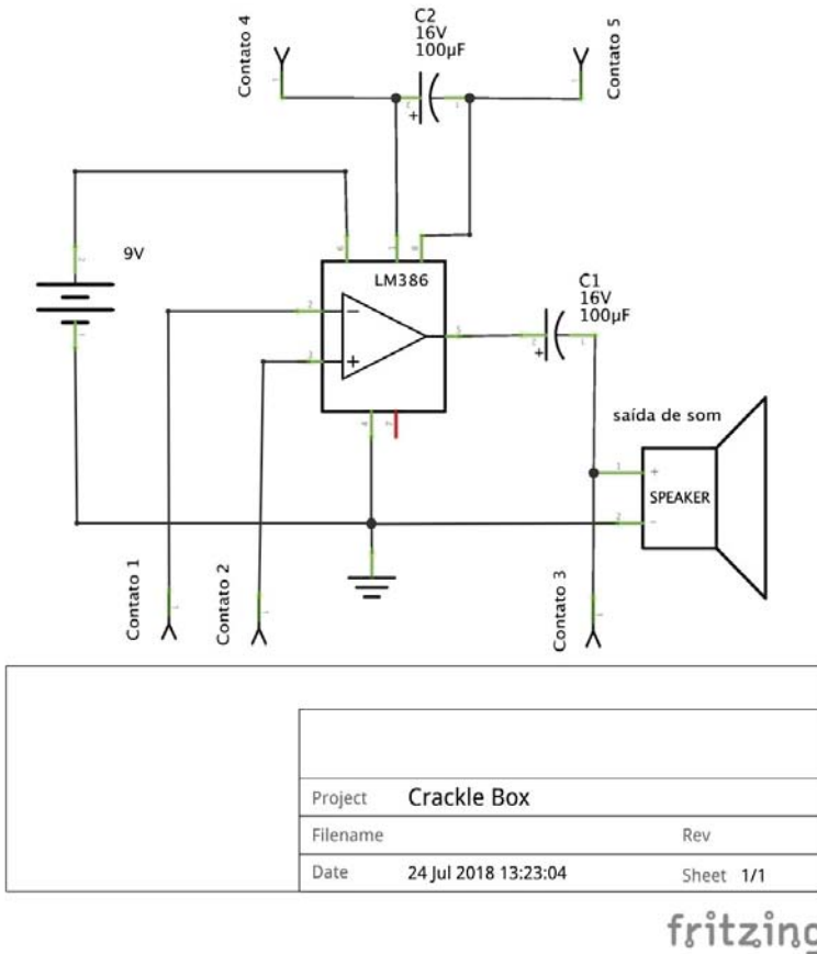
Figura 3 – Circuito Crackle adaptado para nossa oficina
